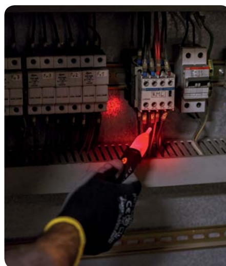
Detección de tensión CA sobre la funda de protección del cable, sin necesidad de tocar partes metálicas
